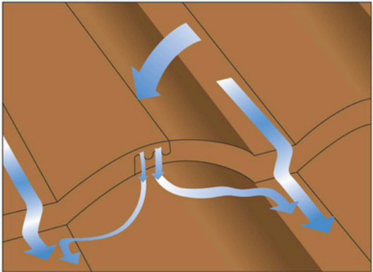
ยอดกันน้ำ 3 ชั้น 2 ร่องลึก ป้องกันน้ำฝนไหลย้อนเข้าใต้หลังคา
